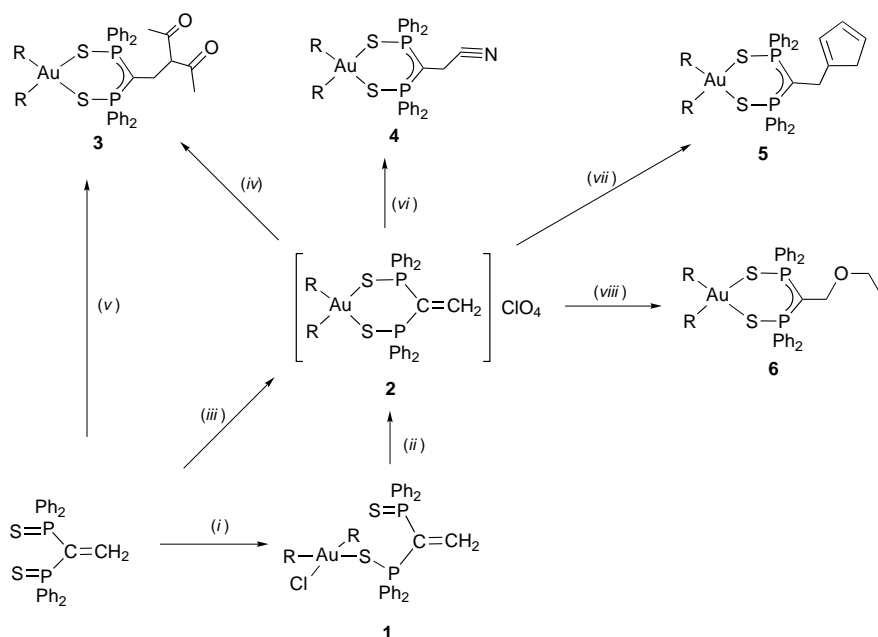
Scheme 3 R = C 6 F 5 . (i) ½ [Au(C 6 F 5 ) 2 (μ-Cl)] 2 ; (ii) AgClO 4 ; (iii) [Au(C 6 F 5 ) 2 (OEt) 2 ]ClO 4 ; (iv) Tl(acac); (v) [Au(C 6 F 5 ) 2 (acac)]; (vi) KCN; (vii) TiCl 5 H 5 ; (viii) NaOEt
